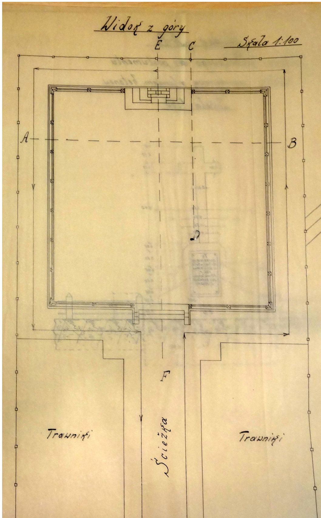
Рис. 6. План обустройства захоронения Fig. 6. Burial arrangement plan
