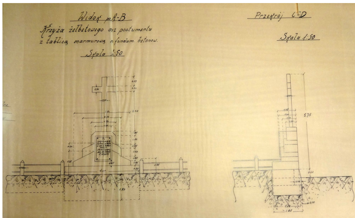
Рис. 7. Схема памятника и креста на могилу повстанцев Fig. 7. Scheme of the monument and the cross on the grave of the rebels
