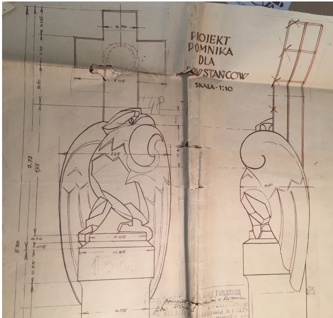
Рис. 2. Схема проекта памятника повстанцам в местечке Куренец Fig. 2. Scheme of the project of the monument to the rebels in the town of Kurenets
