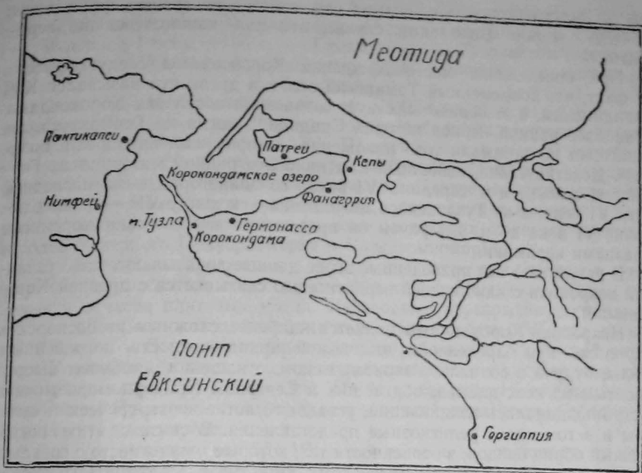
Рис. 24. Карта Таманского полуострова.
